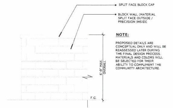
MASONRY WALL SCALE: 1/2"=1'-0" 24
